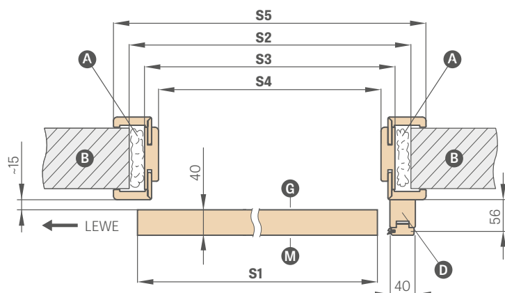
SP1Nz alebo SP1Nb (ľavá verzia líce)
