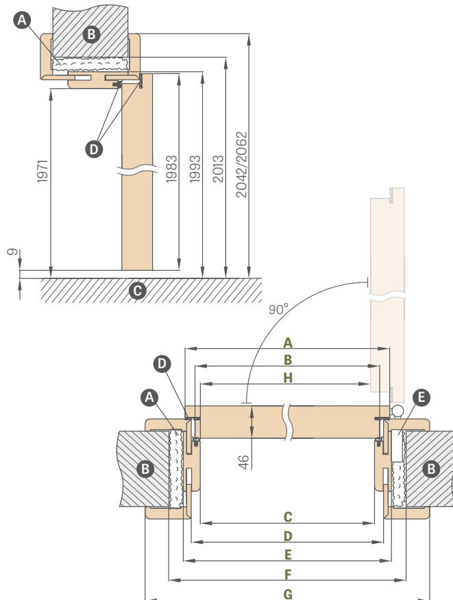
SCHEMA NASTAVITEĽNEJ ZÁRUBNE HERSE SET
