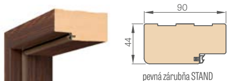
pevná zárubňa STAND
