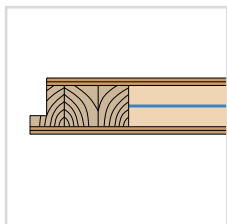
46 mm KRÍDLO spevnené oceľovým plechom
