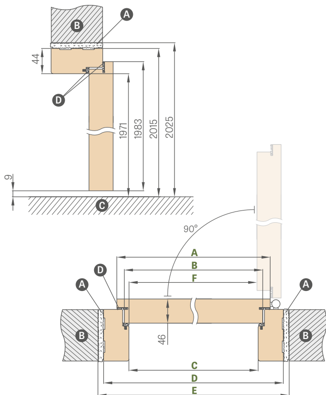
SCHEMA PEVNEJ ZÁRUBNE HERSE SET
